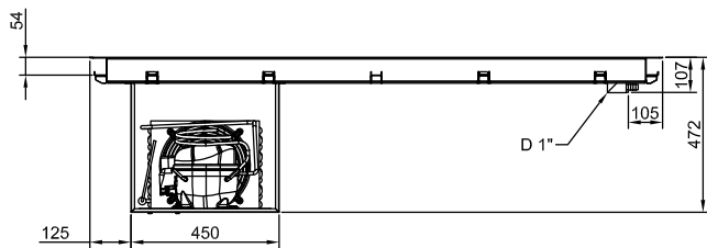
Zij aanzicht
